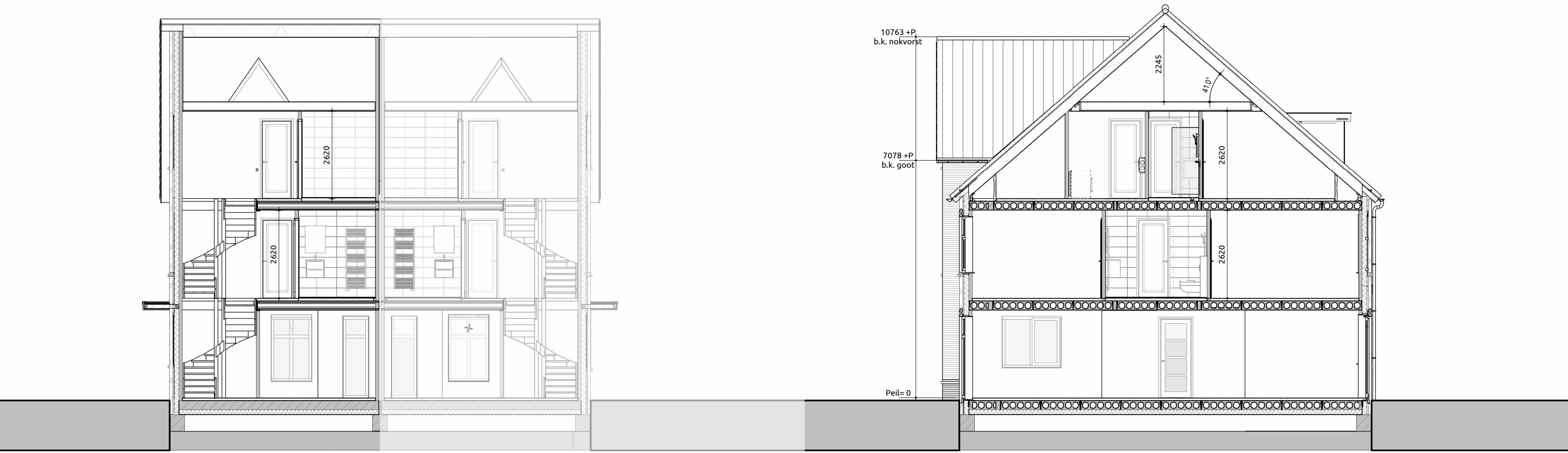
Doorsnede A-A
