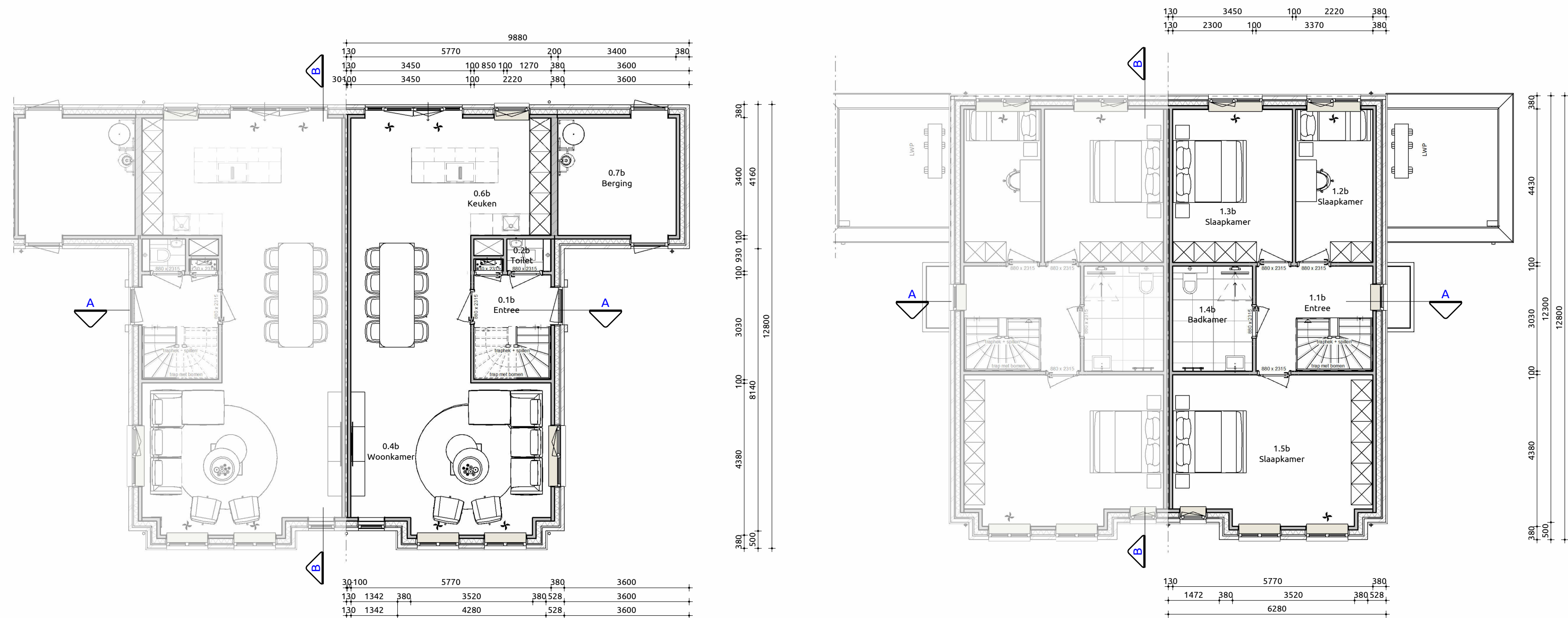
Begane grond
