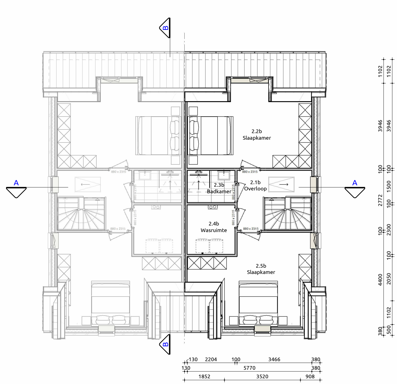
Tweede verdieping
